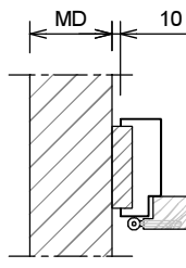
Aansluiting haakse wand
